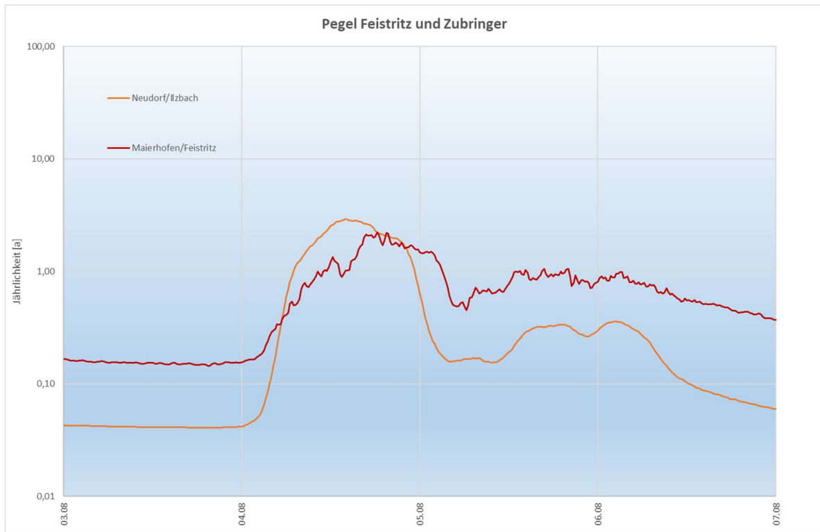
Abbildung 17: Durchflussganglinien normiert auf die Jährlichkeit für die Pegel der Feistritz und deren Zubringer vom 03.08. bis 07.08.2023
