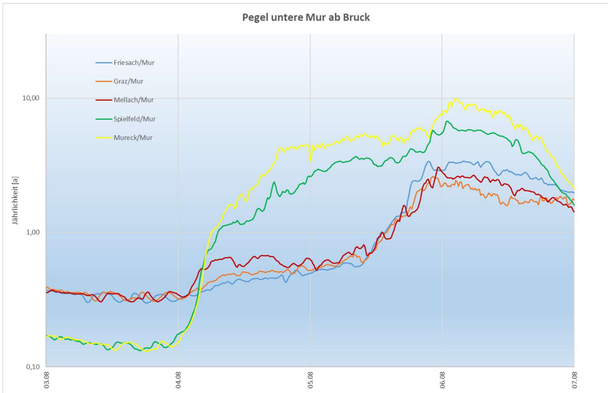
Abbildung 21: Durchflussganglinien normiert auf die Jährlichkeit für die Pegel der unteren Mur ab Bruck vom 03.08. bis 07.08.2023
