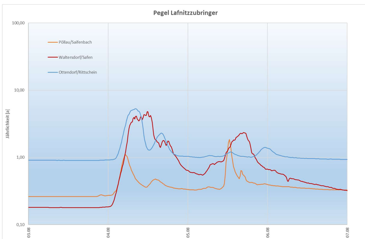
Abbildung 19: Durchflussganglinien normiert auf die Jährlichkeit für die Pegel der Zubringer zur Lafnitz vom 03.08. bis 07.08.2023
