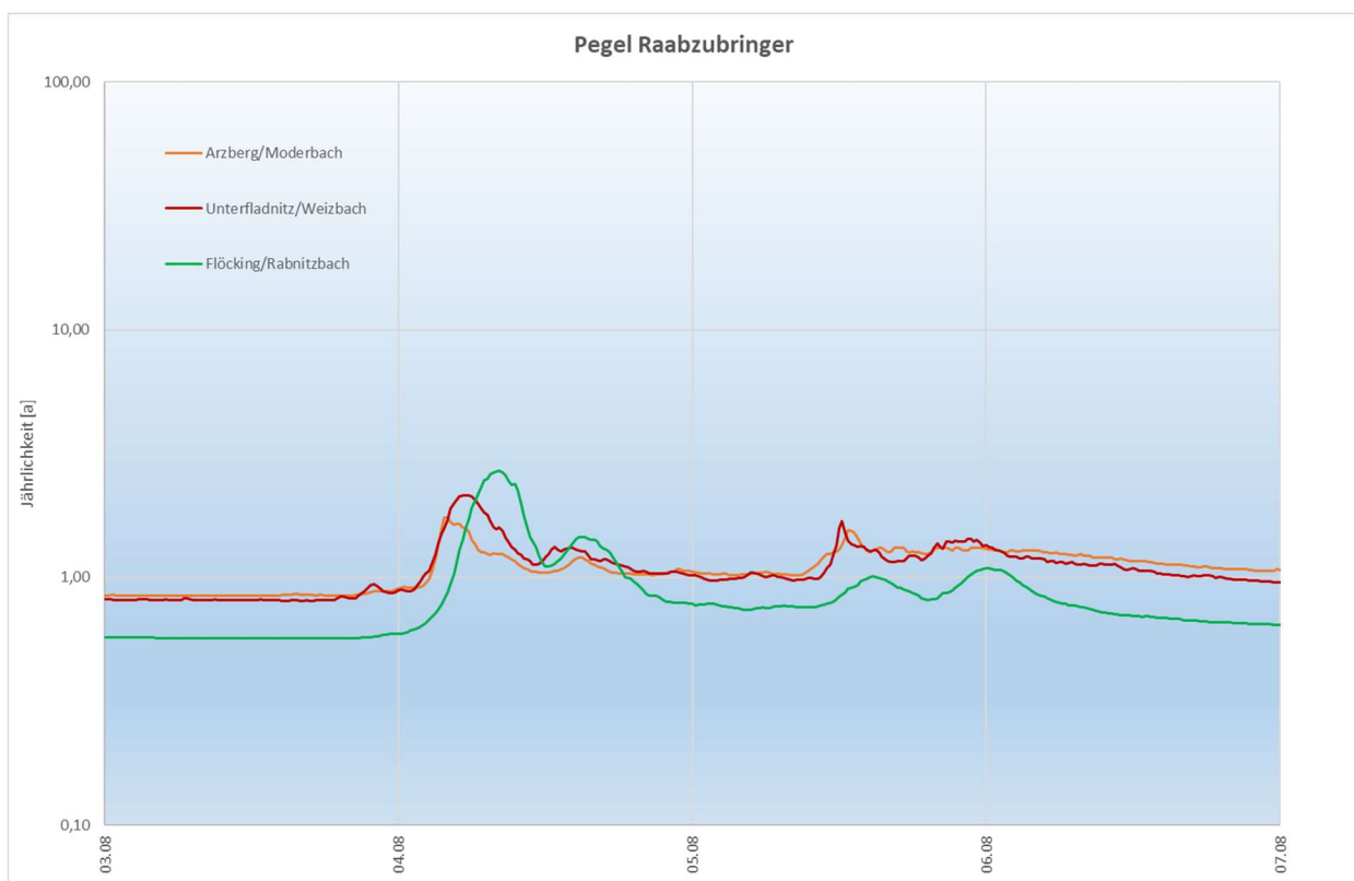
Abbildung 16: Durchflussganglinien normiert auf die Jährlichkeit für die Pegel der Zubringer zur Raab vom 03.08. bis 07.08.2023
