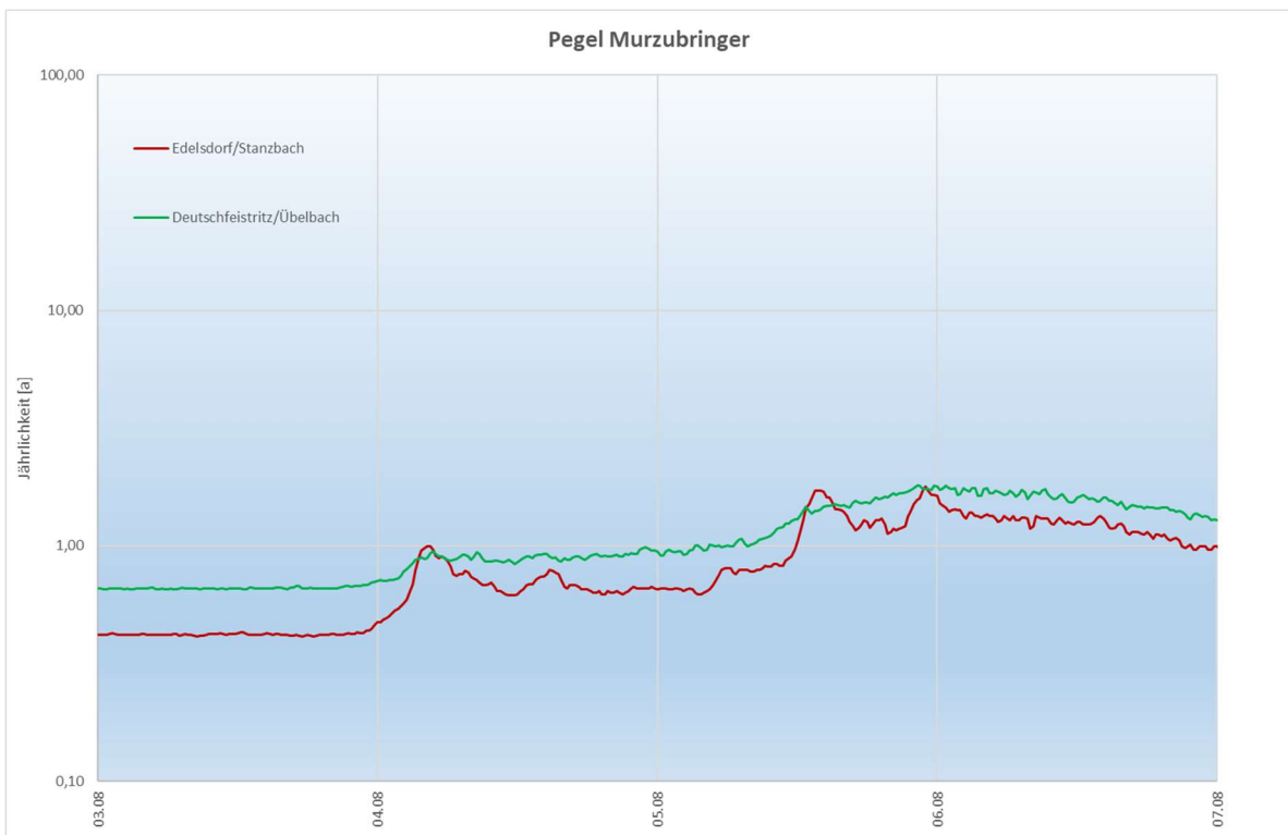
Abbildung 22: Durchflussganglinien normiert auf die Jährlichkeit für die Pegel der Zubringer zur Mur vom 03.08. bis 07.08.2023
