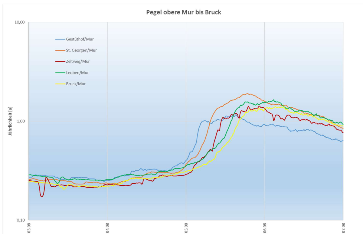
Abbildung 20: Durchflussganglinien normiert auf die Jährlichkeit für die Pegel der oberen Mur bis Bruck vom 03.08. bis 07.08.2023
