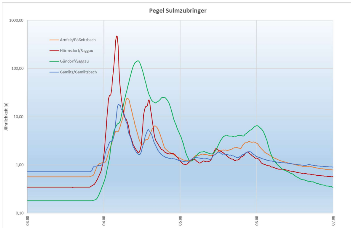
Abbildung 8: Durchflussganglinien normiert auf die Jährlichkeit für die Pegel der Zubringer zur Sulm vom 03.08. bis 07.08.2023
