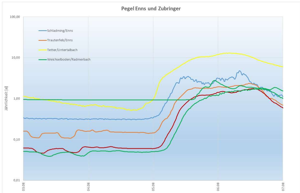
Abbildung 23: Durchflussganglinien normiert auf die Jährlichkeit für die Pegel der Enns und deren Zubringer vom 03.08. bis 07.08.2023
