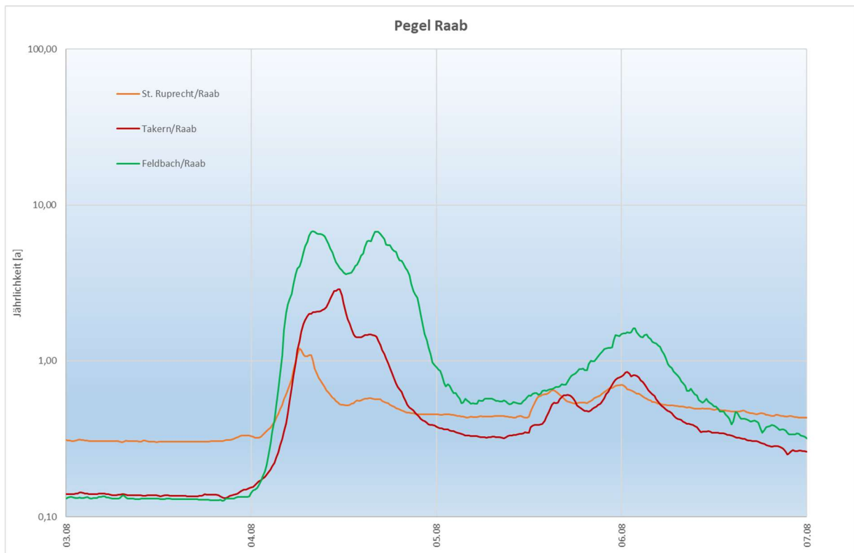
Abbildung 15: Durchflussganglinien normiert auf die Jährlichkeit für die Pegel der Raab vom 03.08. bis 07.08.2023
