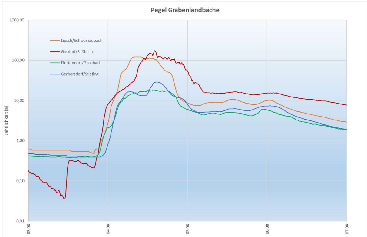
Abbildung 13: Durchflussganglinien normiert auf die Jährlichkeit für die Pegel der Grabenlandbäche vom 03.08. bis 07.08.2023
