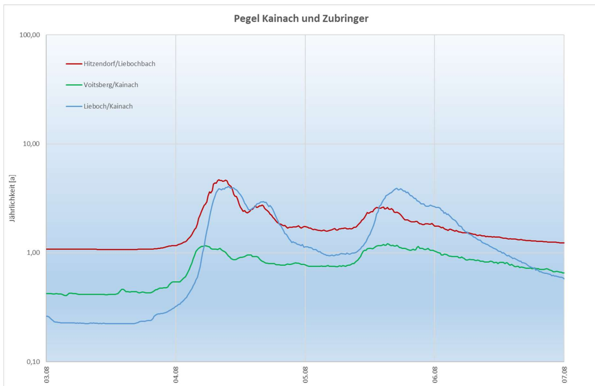
Abbildung 12: Durchflussganglinien normiert auf die Jährlichkeit für die Pegel der Kainach und deren Zubringer vom 03.08. bis 07.08.2023
