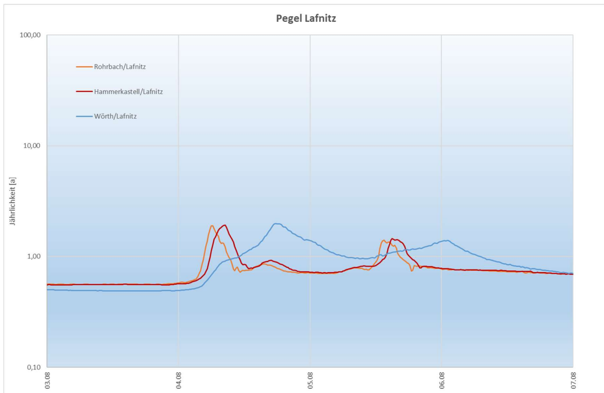
Abbildung 18: Durchflussganglinien normiert auf die Jährlichkeit für die Pegel der Lafnitz vom 03.08. bis 07.08.2023
