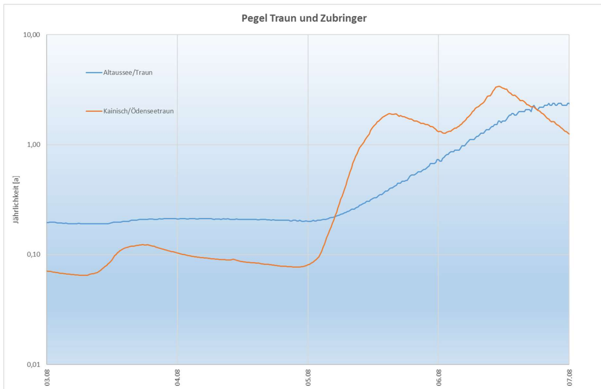
Abbildung 24: Durchflussganglinien normiert auf die Jährlichkeit für die Pegel der Zubringer zur Traun vom 03.08. bis 07.08.2023
