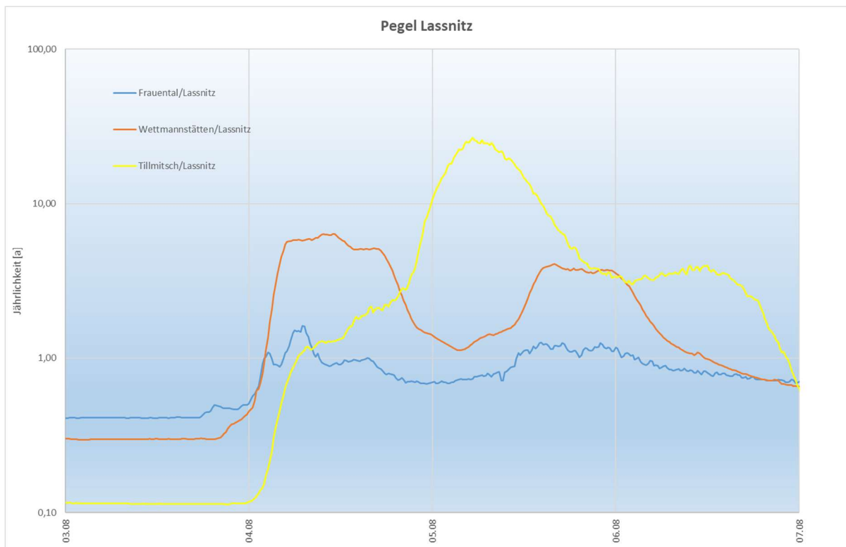
Abbildung 10: Durchflussganglinien normiert auf die Jährlichkeit für die Pegel der Lassnitz vom 03.08. bis 07.08.2023
