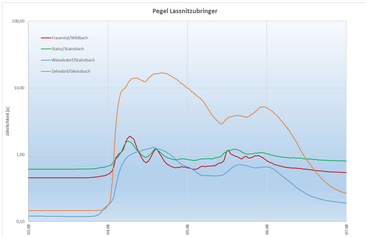
Abbildung 11: Durchflussganglinien normiert auf die Jährlichkeit für die Pegel der Zubringer zur Lassnitz vom 03.08. bis 07.08.2023
