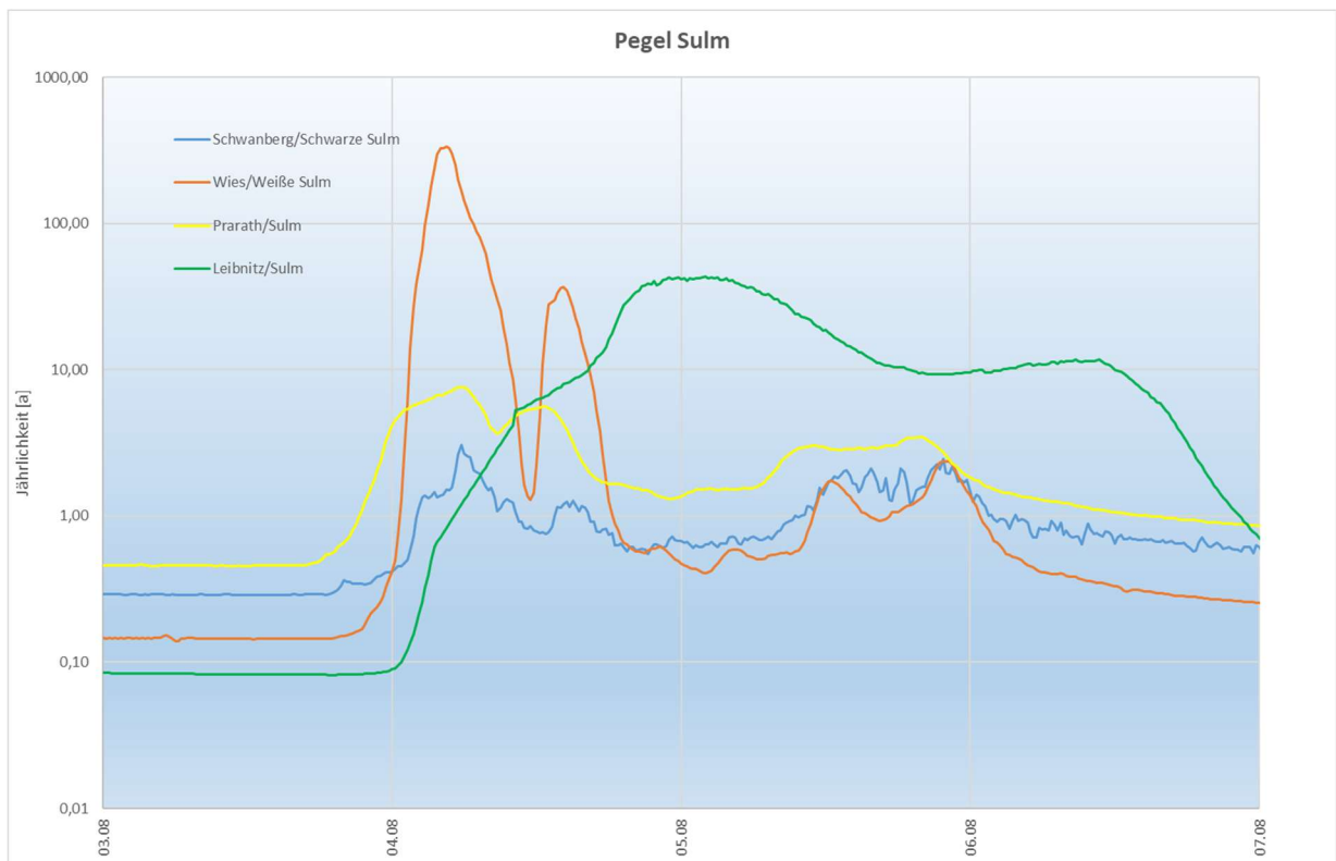
Abbildung 6: Durchflussganglinien normiert auf die Jährlichkeit für die Pegel der Sulm vom 03.08. bis 07.08.2023
